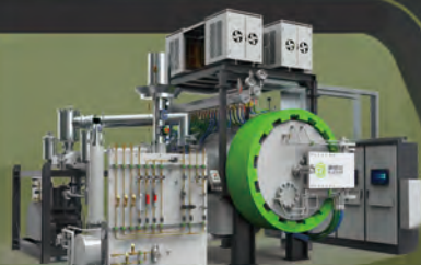
压力烧结炉
